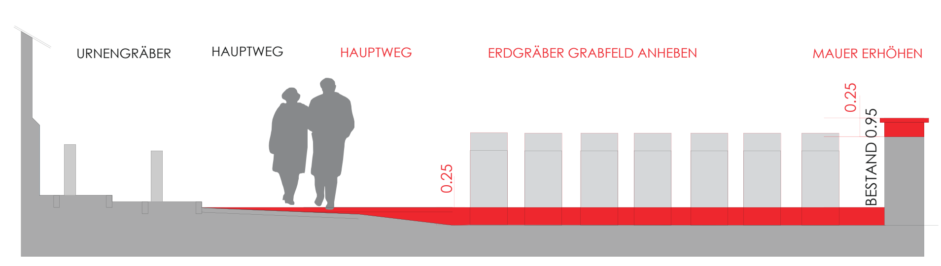
SCHNITTANSICHT B M. 1 : 50
