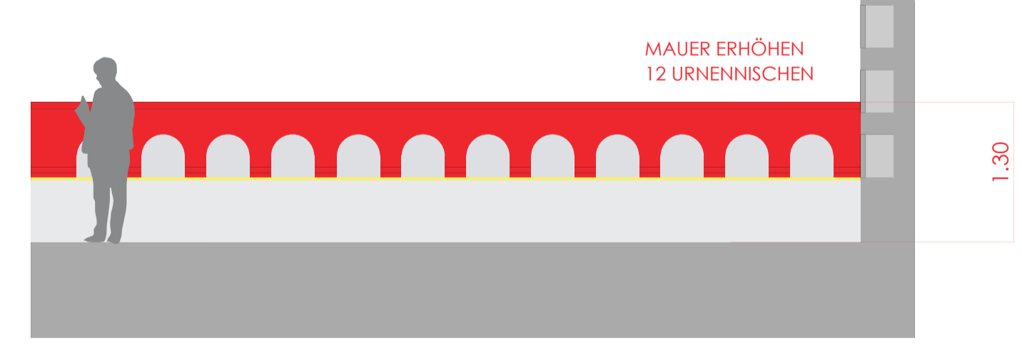
SCHNITTANSICHT A M. 1 : 50
