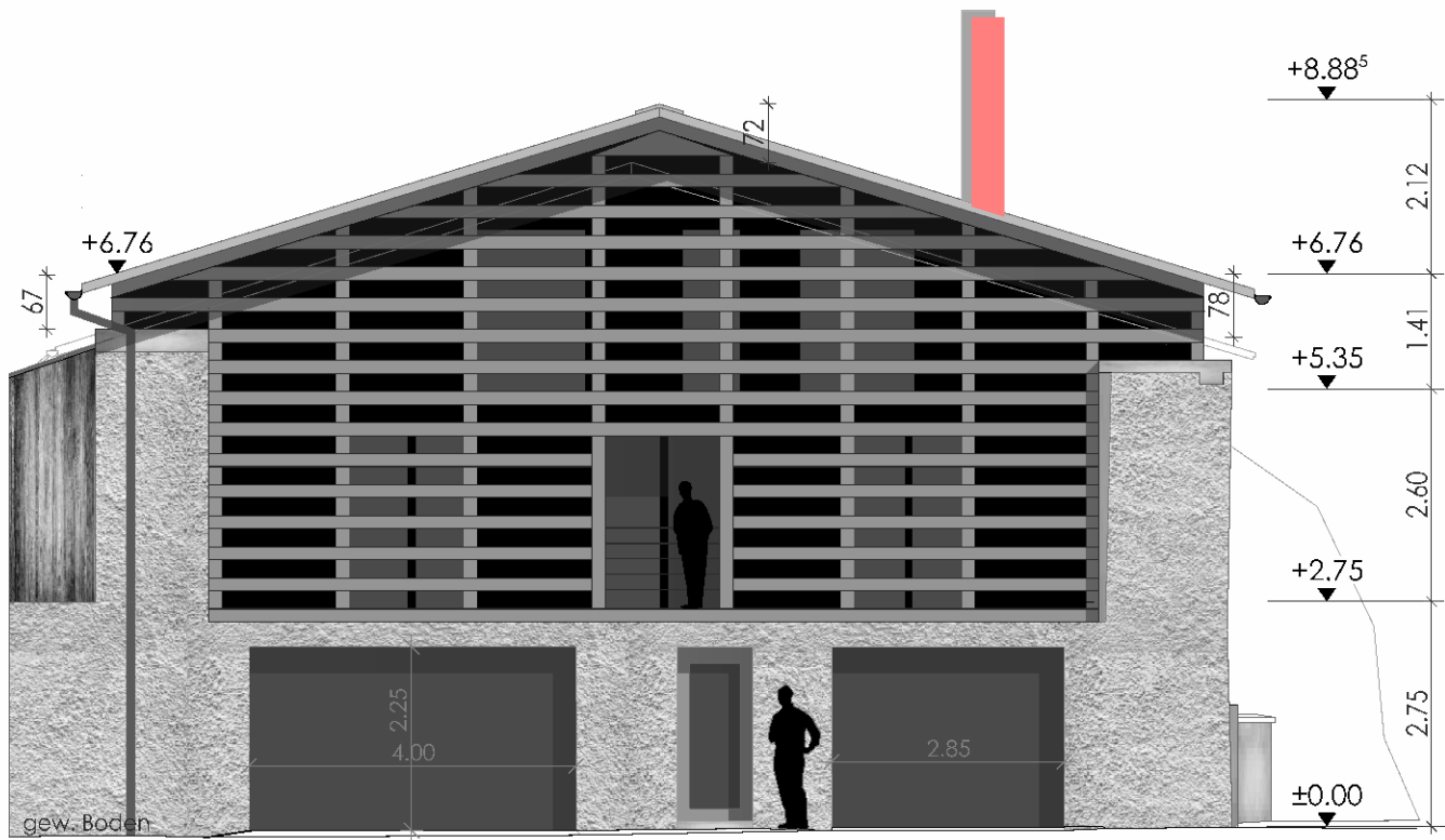
Nordwest Fassade
