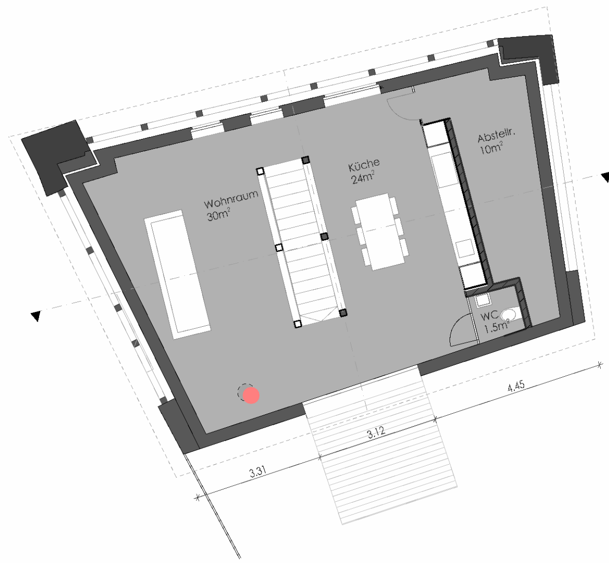
Dachgeschoss
