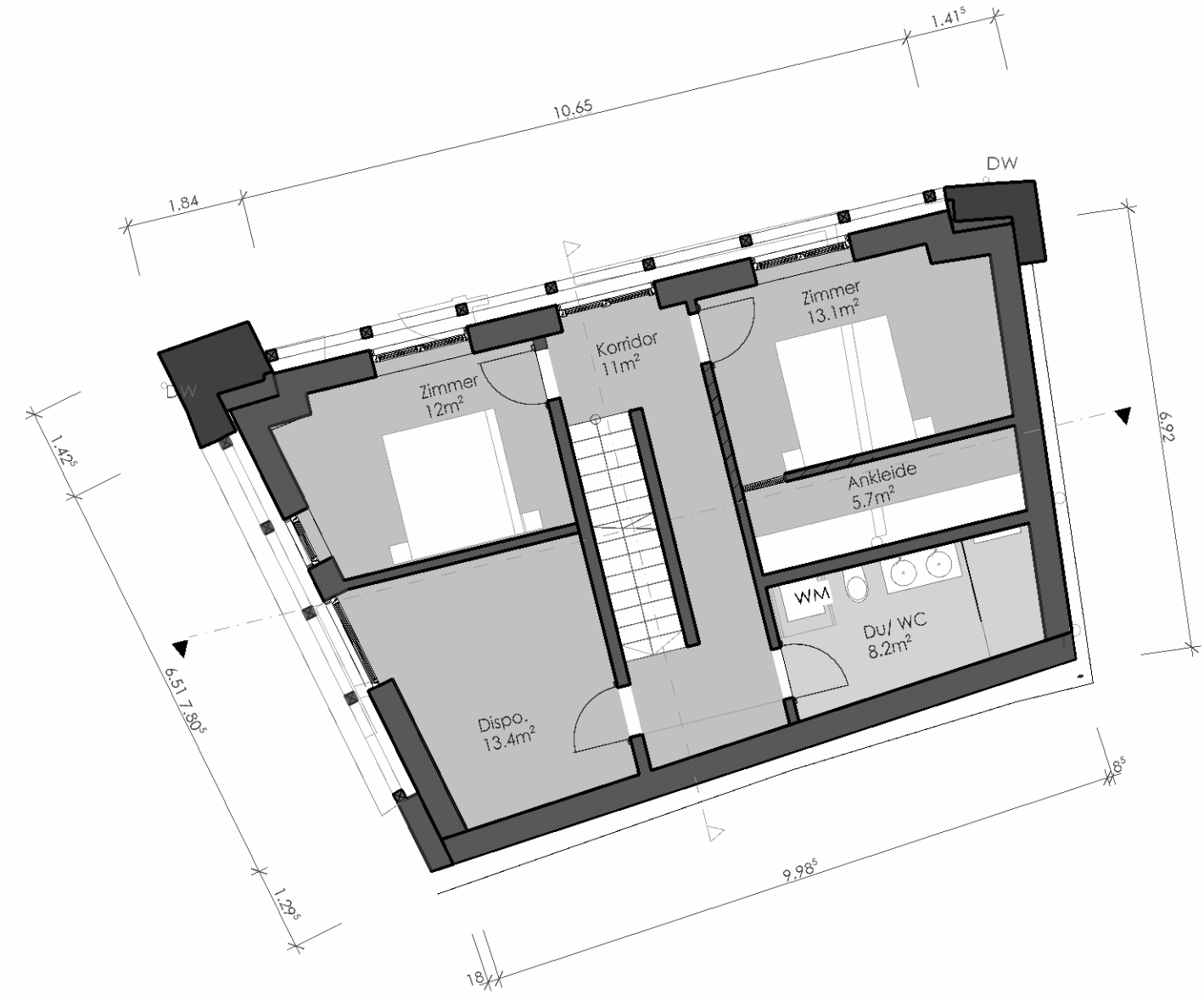
Dachgeschoss
