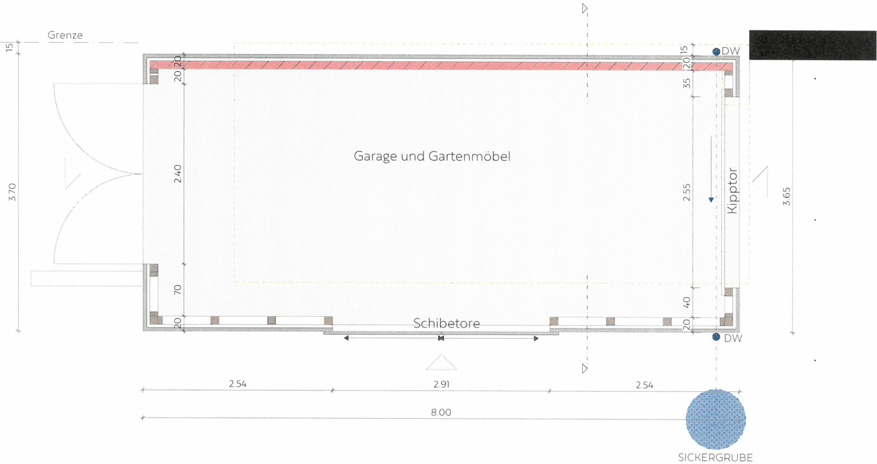
Grundriss
