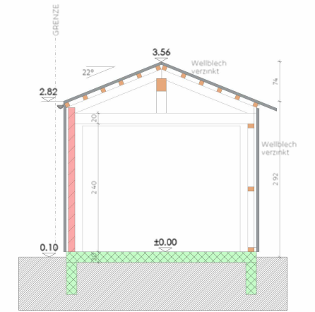
Querschnitt
