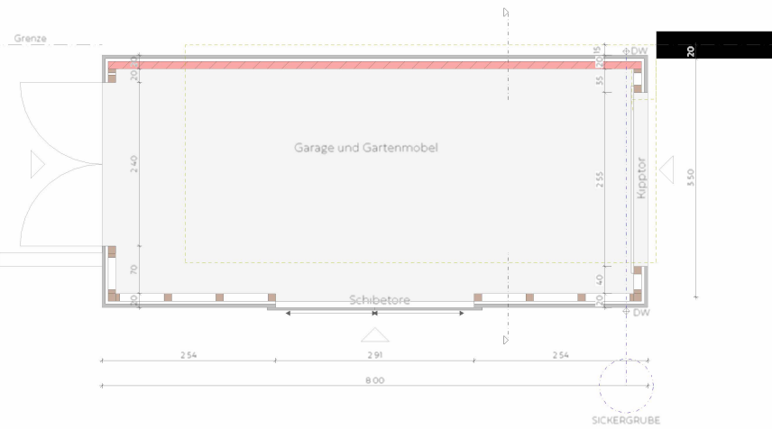
Grundriss
